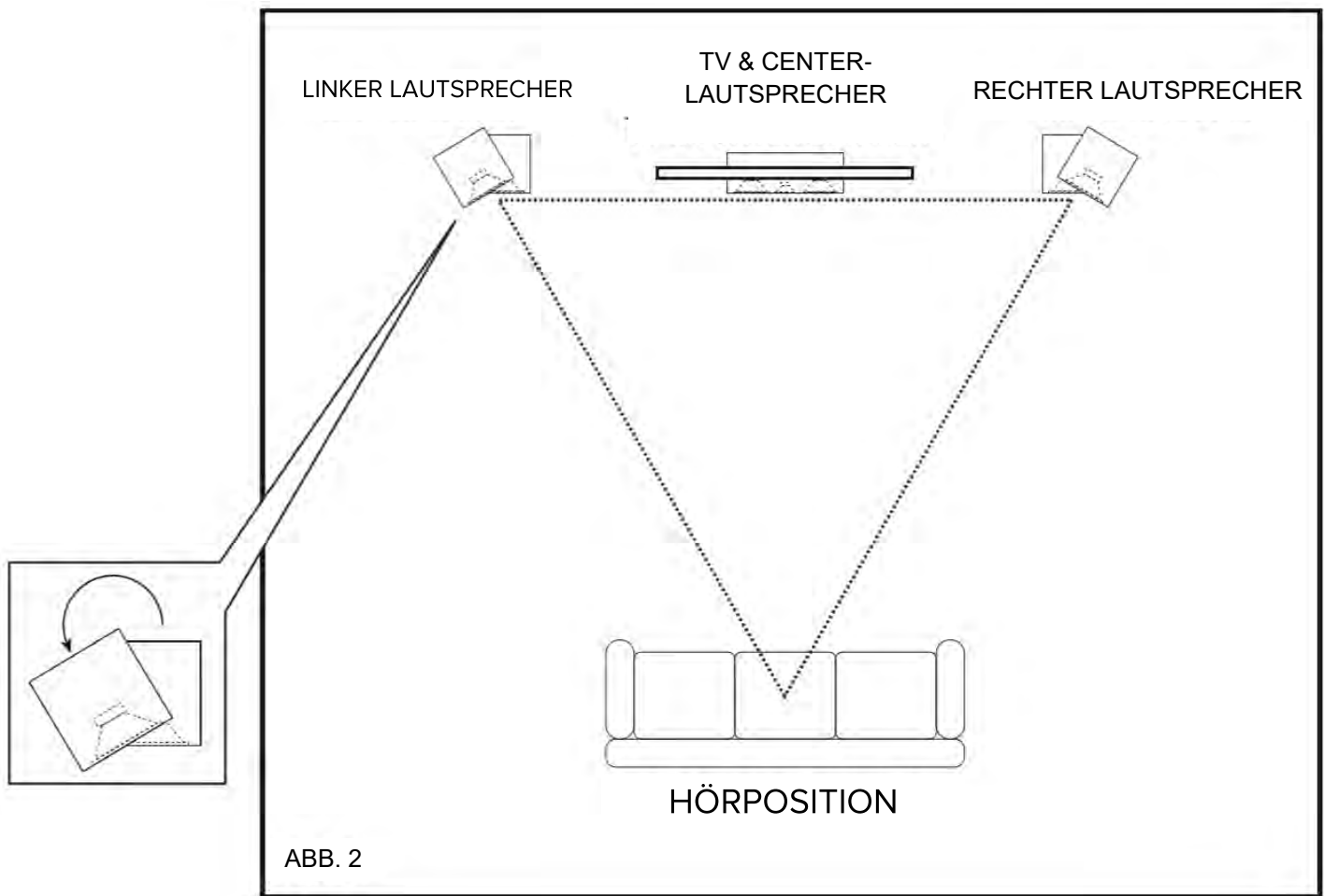
2-KANAL-STEREO-ANORDNUNG
