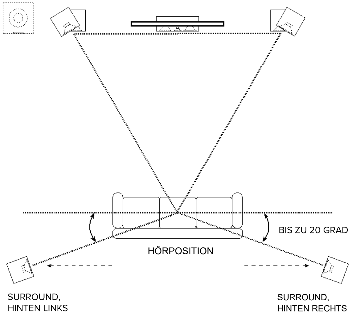
5.1-KANAL-SURROUND-KONFIGURATION
